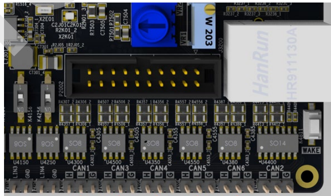
图 5. CAN 接口
