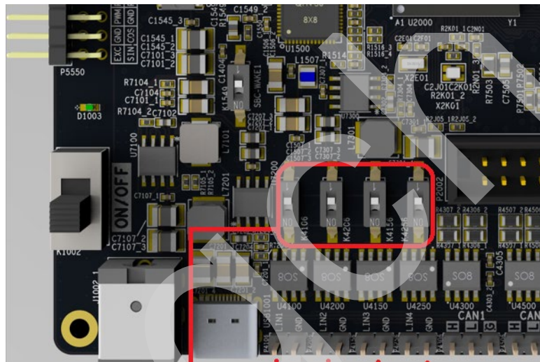
图 4. LIN 接口
